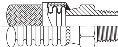
NPT/BSPT/BSPP Male w/Hex Nut
